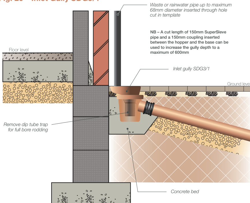
Fig. 20 – Inlet Gully SDG3/1
