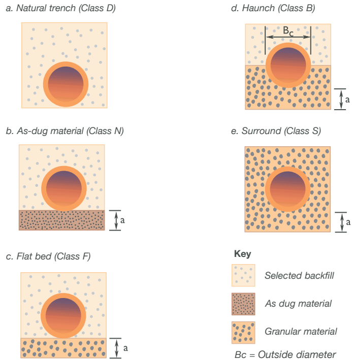
Fig. 5 – Bedding
